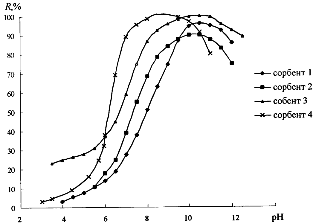
Рис. 27. Зависимость степени сорбции ( R, \% ) Cd (II) сорбентами 1-4 от pH среды
