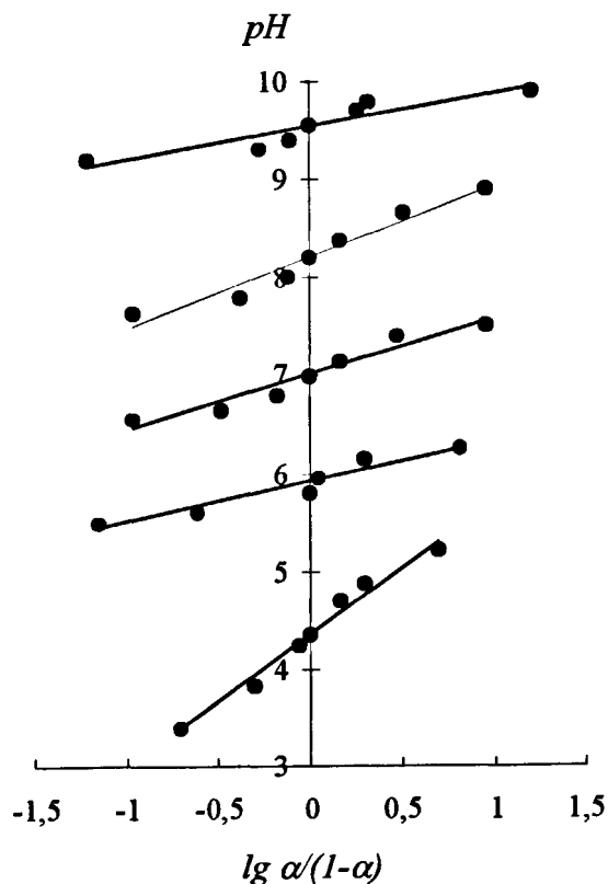
Рис. 13 . Графическое определение констант ионизации ( pK_{\text{ион}} ) сорбента 9 полистирол-2-окси-азо-2'-окси, 3'-карбокси, 5'-бензолсульфонокислота
