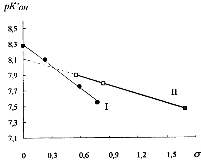
Рис. 55. Корреляции между кислотно-основными свойствами моно-(I) и дизамещенных (II) хелатообразующих сорбентов ( pK'_{OH} ) и константами Гаммета \sigma
