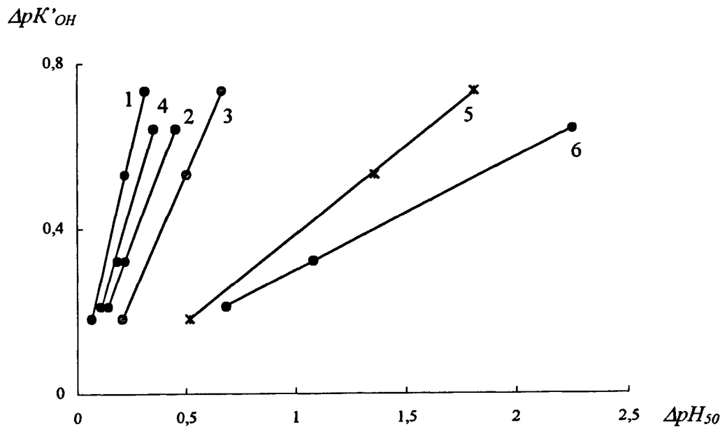
Рис. 57. Корреляции между кислотно-основными свойствами моно- и дизамещенных хелатообразующих сорбентов и pH_{50} сорбции кобальта (1, 2), никеля (3, 4) и кадмия (5,6) соответственно
