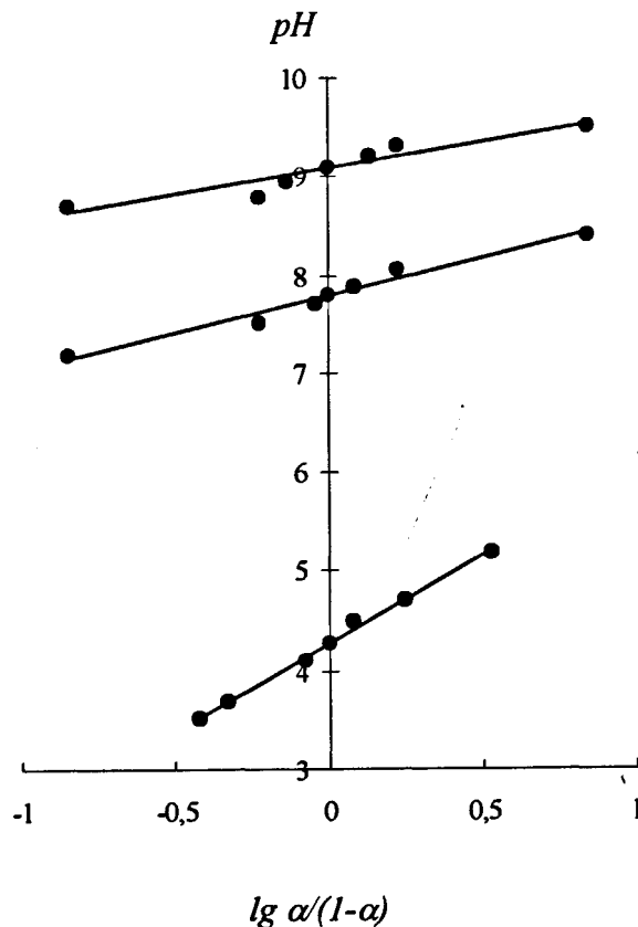
Рис. 10. Графическое определение констант ионизации ( pK_{\text{ион}} ) сорбента 6 полистирол-2-окси-азо-2'-окси, 3', 5'-бензолдисульфокислота
