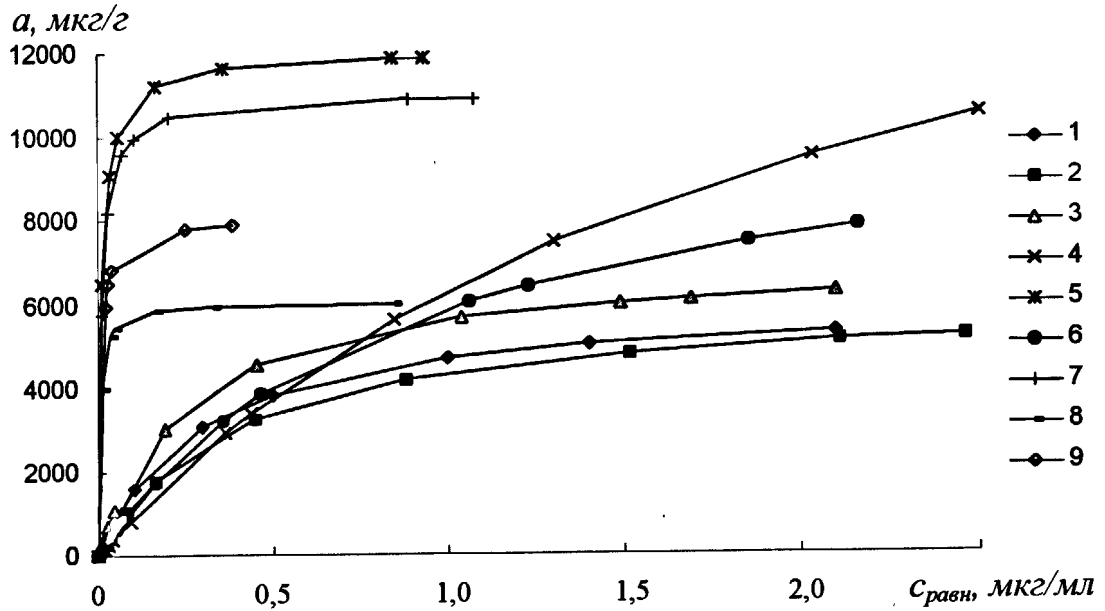
Рис.36. Изотермы сорбции ионов кадмия(II) на сорбентах 1-9 ( m(\text{сорбента})=20 мг, V(\text{раствора})=20 мл, t=20^{\circ}\text{C} , pH 6,8)
