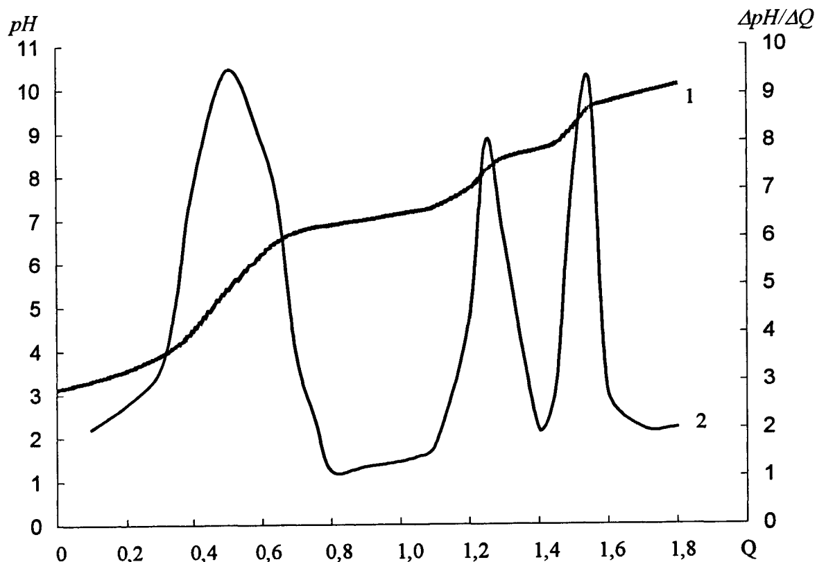
Рис. 4. Интегральная (1) и дифференциальная (2) кривые титрования сорбента полистирол-2-окси-азо-2'-окси, 5'-хлор, 3'-бензолсульфоуксислота
