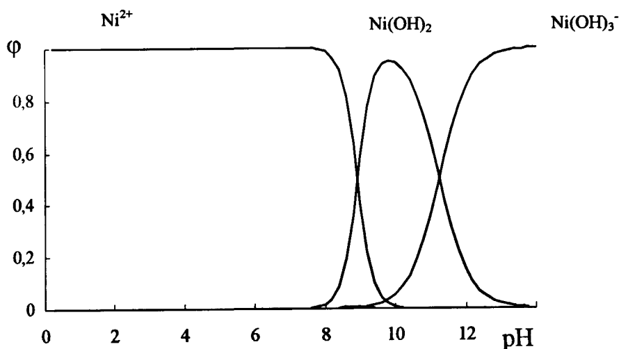
Рис. 2. Кривые распределения \text{Ni}^{2+} и его гидроксоформ в зависимости от pH раствора ( \text{pK}_{\text{r1}} 10,97 ; \text{pK}_{\text{r2}} 6,87 ; \text{pK}_{\text{r3}} 11,25 )
