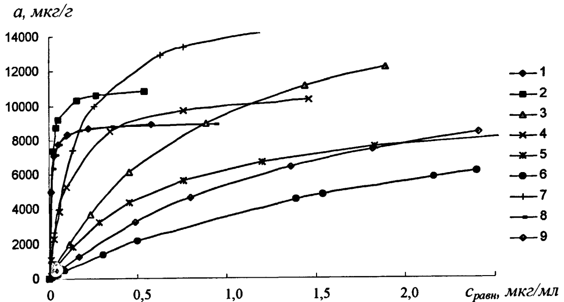
Рис.34. Изотермы сорбции ионов кобальта(II) на сорбентах 1-9 ( m(\text{сорбента})=20 \text{ мг} , V(\text{раствора})=20 \text{ мл} , t=20^\circ\text{C} , pH \text{ 6,8} )
