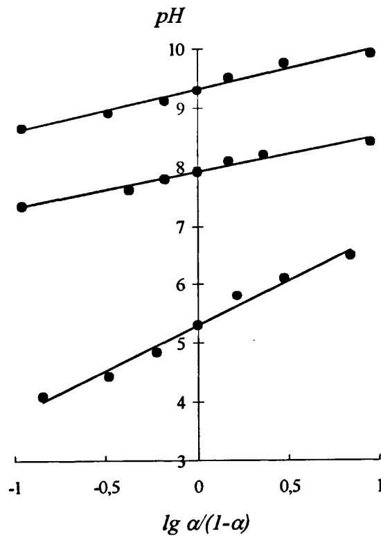
Рис. 9. Графическое определение констант ионизации ( pK_{\text{ион}} ) сорбента 5 полистирол-2-окси-азо-2'-окси, 5'-хлор, 3'-бензолсульфоукислота
