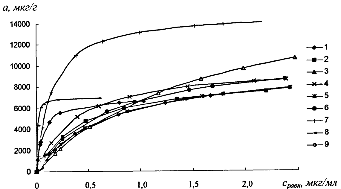
Рис.35. Изотермы сорбции ионов никеля(II) на сорбентах 1-9 ( m(\text{сорбента})=20 \text{ мг} , V(\text{раствора})=20 \text{ мл} , t=20^\circ\text{C} , pH \text{ 6,8} )
