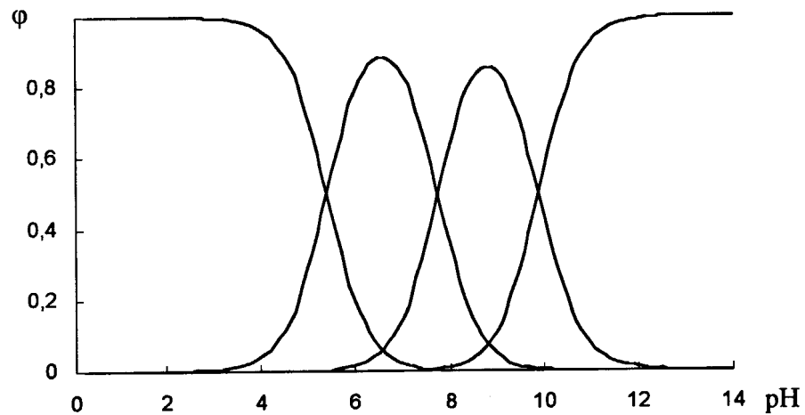
Рис. 16. Кривые распределения равновесных форм сорбента 3 в зависимости от pH среды ( \mu=1 )
