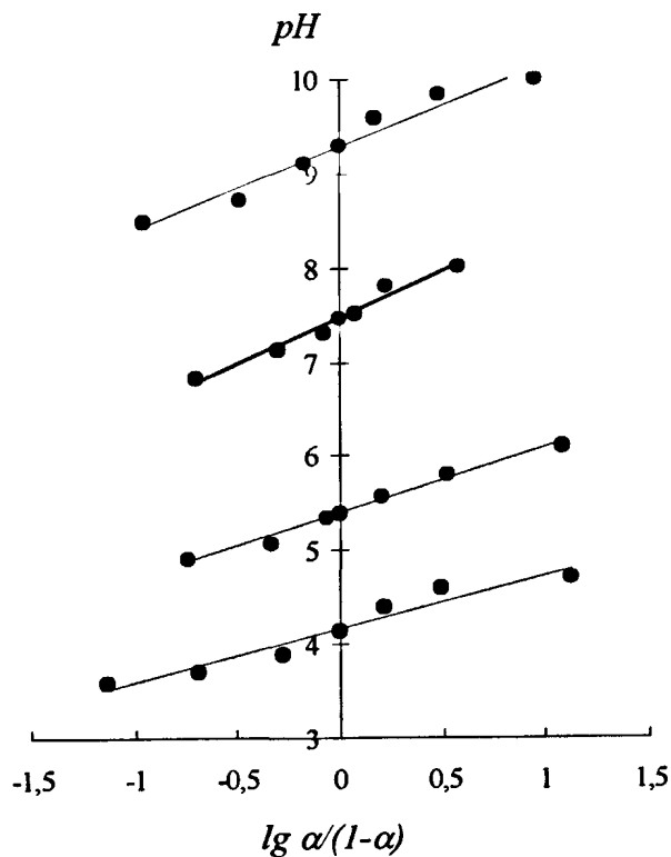
Рис. 11. Графическое определение констант ионизации ( pK_{\text{ион}} ) сорбента 7 полистирол-2-окси-азо-2'-окси, 5'-нитро, 3'-бензолсульфоукислота
