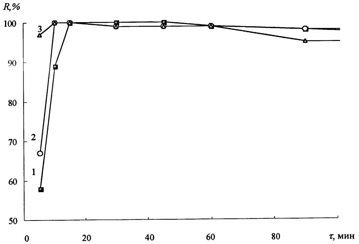
Рис.29. Зависимость сорбции никеля от времени и температуры сорбентом 7 (1- при 20°C, 2 - при 40 °С, 3 - при 60 °С)
