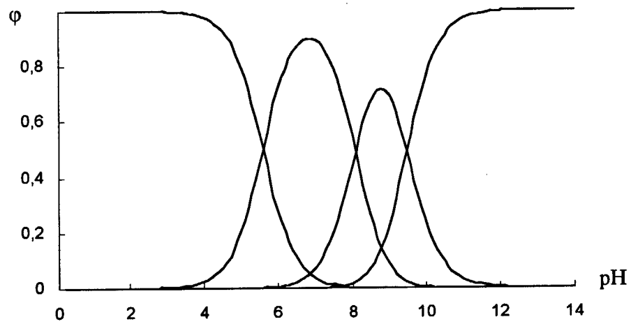
Рис. 15. Кривые распределения равновесных форм сорбента 2 в зависимости от pH среды ( \mu=1 )
