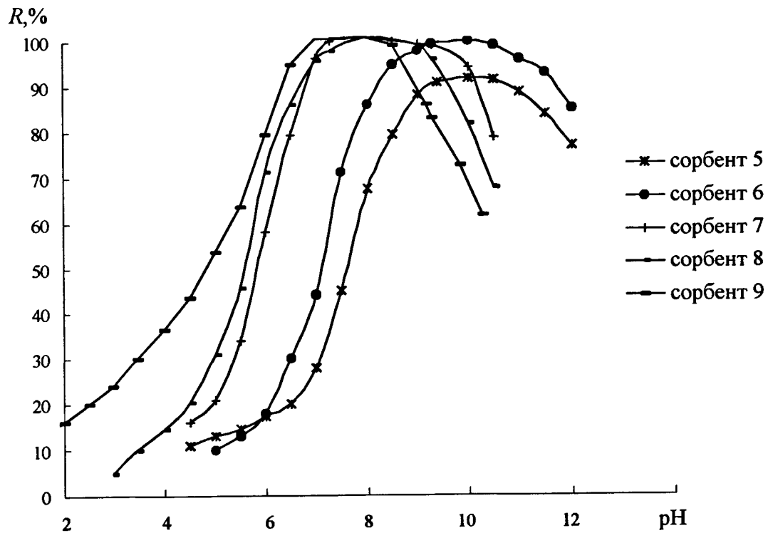
Рис. 28. Зависимость степени сорбции ( R, \% ) Cd (II) сорбентами 5-9 от pH среды
